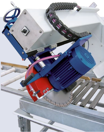
0-45° (Gehrung)
