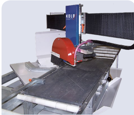
-45°/0°/+45° (Schrägschnitt)
