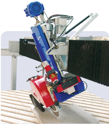
Tilting device 0° - 45° (mitre cutting) (optional)
